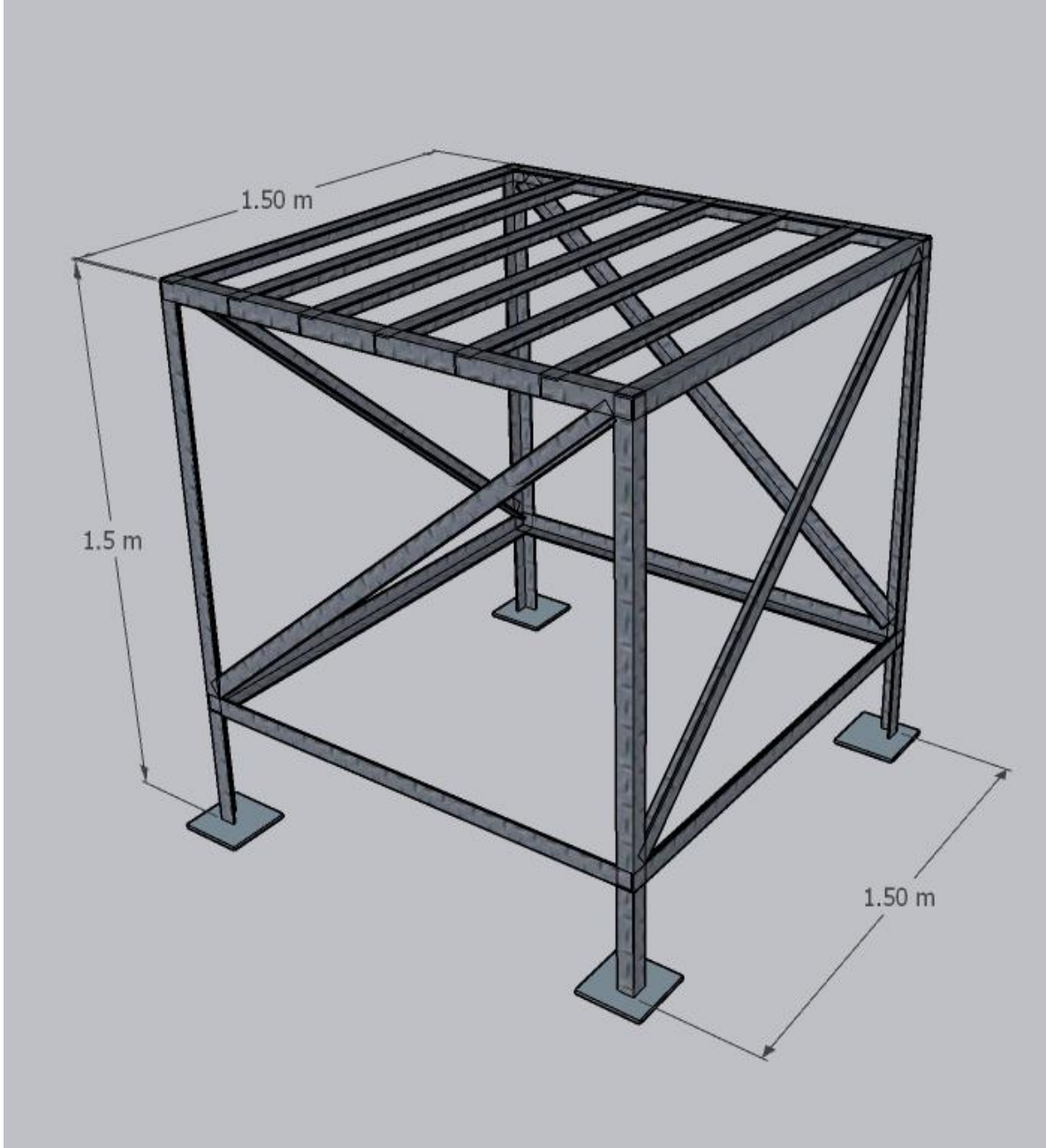
قاعدة خزان الماء
